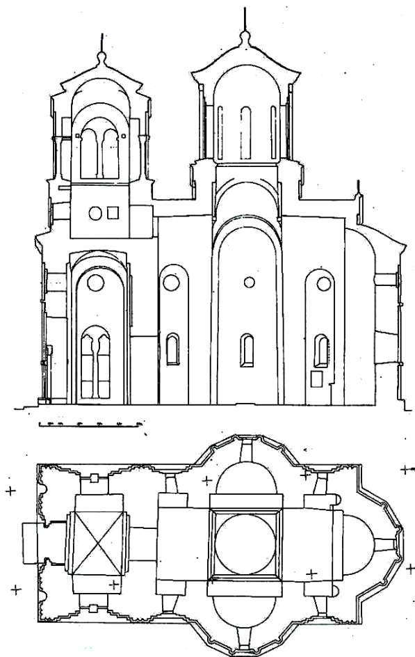
Lazarica: presek, osnova i pogled sa jugoistoka
